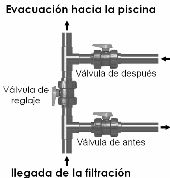
Esquema By-pass
